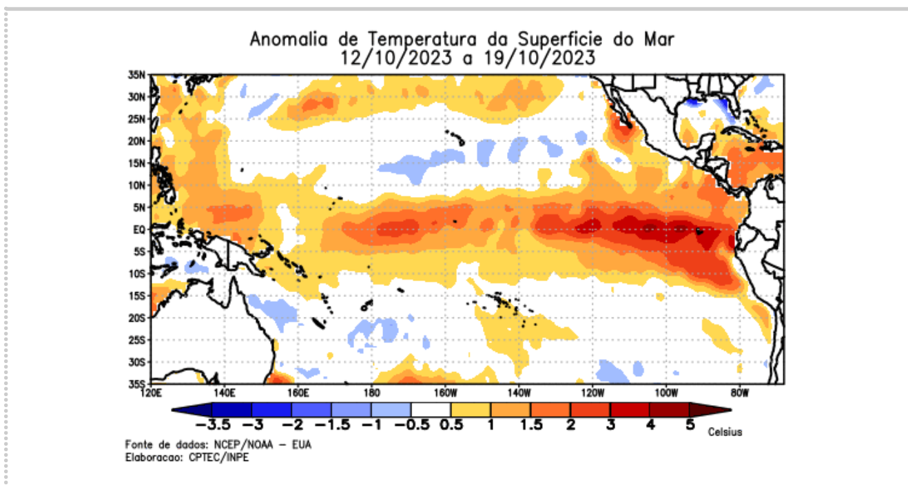
Figura 1.2: Anomalia da temperatura da superfície do mar na região do Pacífico durante o período de 12 e 19 de outubro de 2023.
