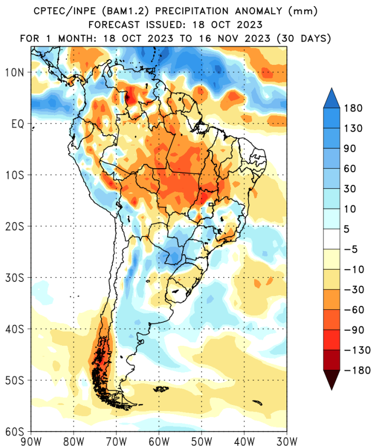
Figura 2.1: Previsão de anomalia de precipitação para o período de 1 mês (de 18 de outubro a 16 de novembro de 2023) produzida no dia 18 de outubro de 2023 com o modelo global atmosférico do CPTEC/INPE (BAM-1.2).
