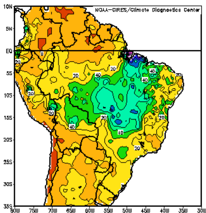
Figura 11 - Totais de precipitação ( \text{cm.mes}^{-1} ) para fevereiro de 1980. Fonte de dados: Udel/CDC/CIRES/NOAA.
