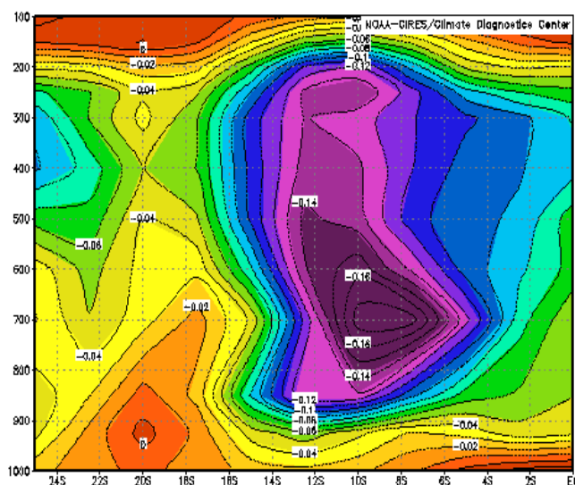
Figura 5 - Seção de \omega ( \text{hPa s}^{-1} ) ao longo de 45°W para o dia 8 de fevereiro de 1980.
