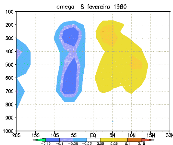
Figura 3 - Seção de \omega ( \text{hPa s}^{-1} ) ao longo de 60°W para o dia 8 de fevereiro de 1980
