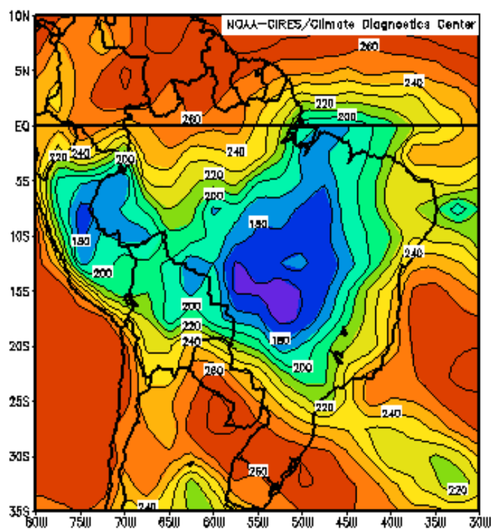
Figura 10 - Radiação de onda longa emergente média ( \text{Wm}^{-2} ), período 7 a 16 de fevereiro de 1980. Fonte de dados: CDC/CIRES/NOAA.
